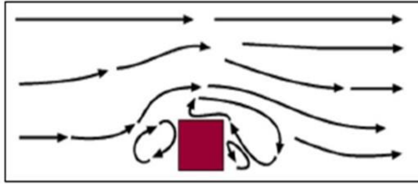
Şekil 3.8 : Bir engel etrafında rüzgar akışı
